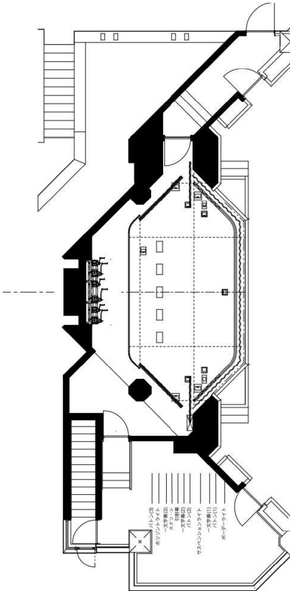
岩国市民文化会館小ホール 平面図
